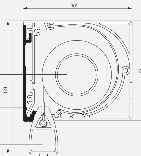
Grote cassette, hoekig
