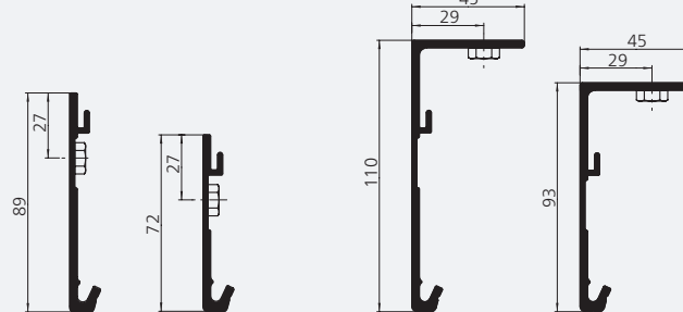
Muurconsole voor 75 en 92 mm cassettes
