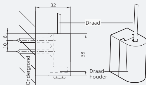
Muur- en dagkantmontage
