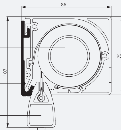
Kleine cassette, hoekig
