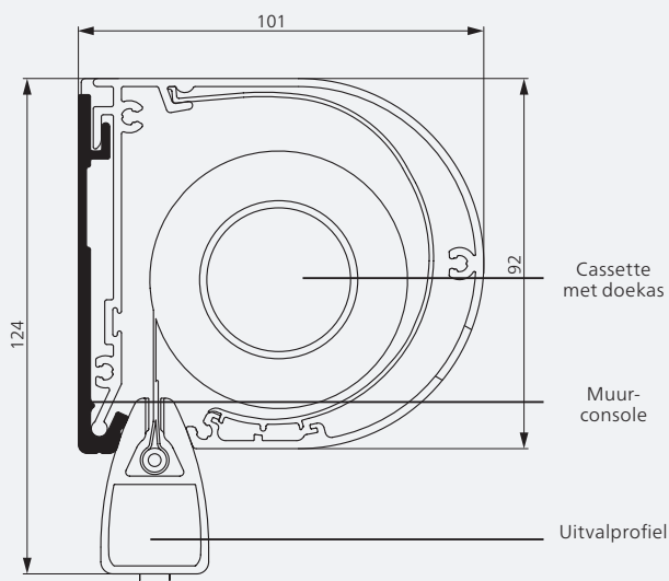
Grote cassette, rond
