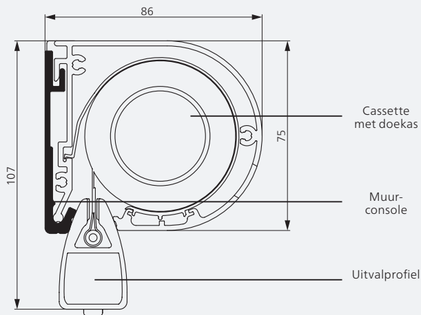
Grote cassette, rond
